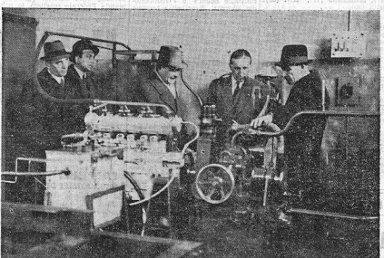
Il nuovo motore 6 cilindri della Maserati è sul banco di prova. Assistono i fratelli Mazzotti e il conte Carlo Felice Trossi.
